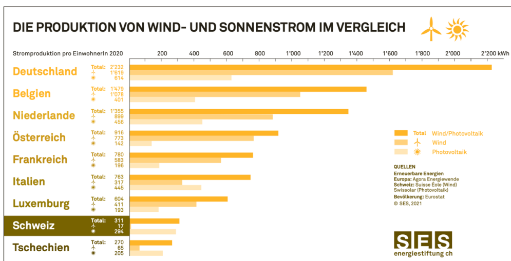
Abbildung 8: Pro-Kopf-Produktion von Solar- und Windstrom in der Schweiz im Vergleich mit 8 umliegenden Ländern im 2020. Daten: EurObserv'ER, Agora Energiewende, Suisse Eole, Swissolar, Eurostat, Bundesamt für Energie, eigene Berechnung. Eigene Darstellung © SES.
