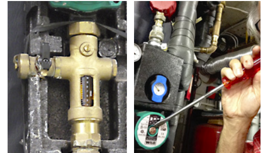
Links: Durchflussmesser mit Schwimmer hinter Skalglass. Rechts: Trick zum besseren Hören der UWP-Geräusche
